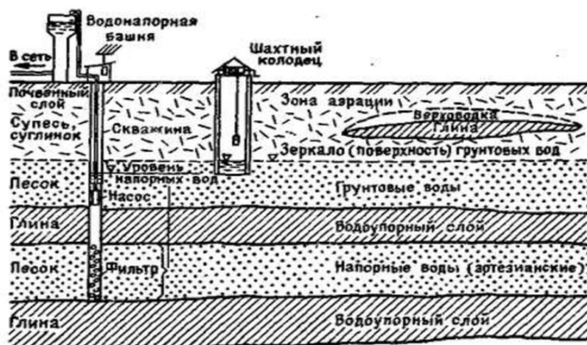
Рис. 2. Схема глубинного расположения подземных водных источников
